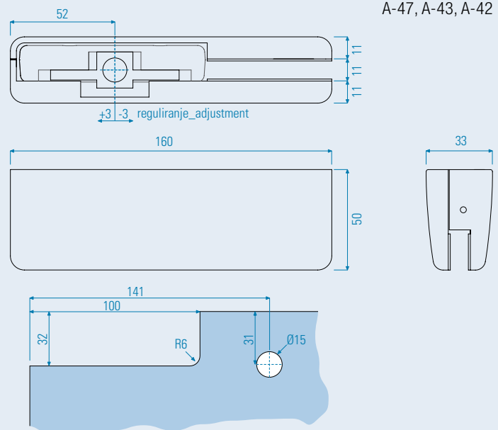
zgornji tečaj krilnih vrat_upper door hinge
