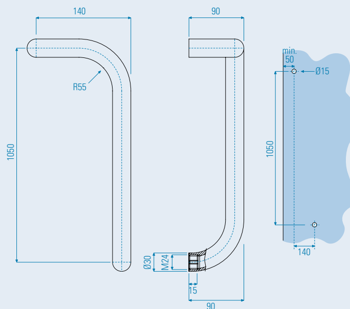
cevasti ročaj_tubular handle
