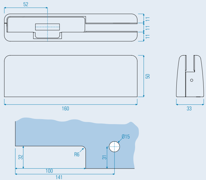
spodnji tečaj krilnih vrat_lower door hinge
