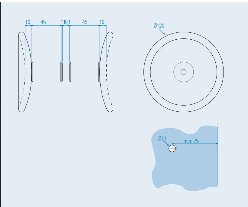
okrogli ročaj fi 12cm_doorknob fi 12cm
