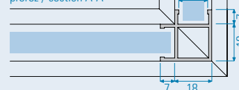
prerez / section A-A
